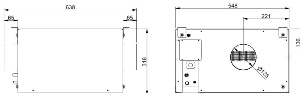
Unité intérieure
